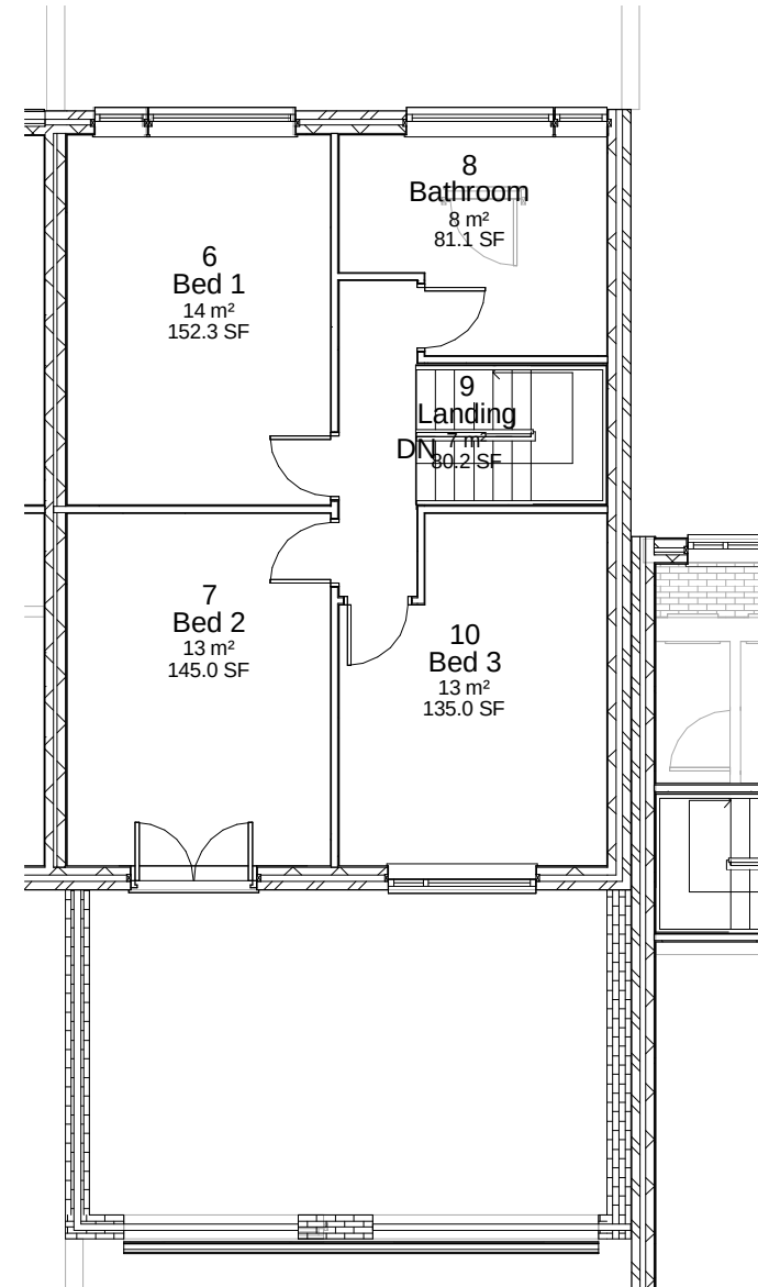
2 Level 1 - 40A 1 : 100
