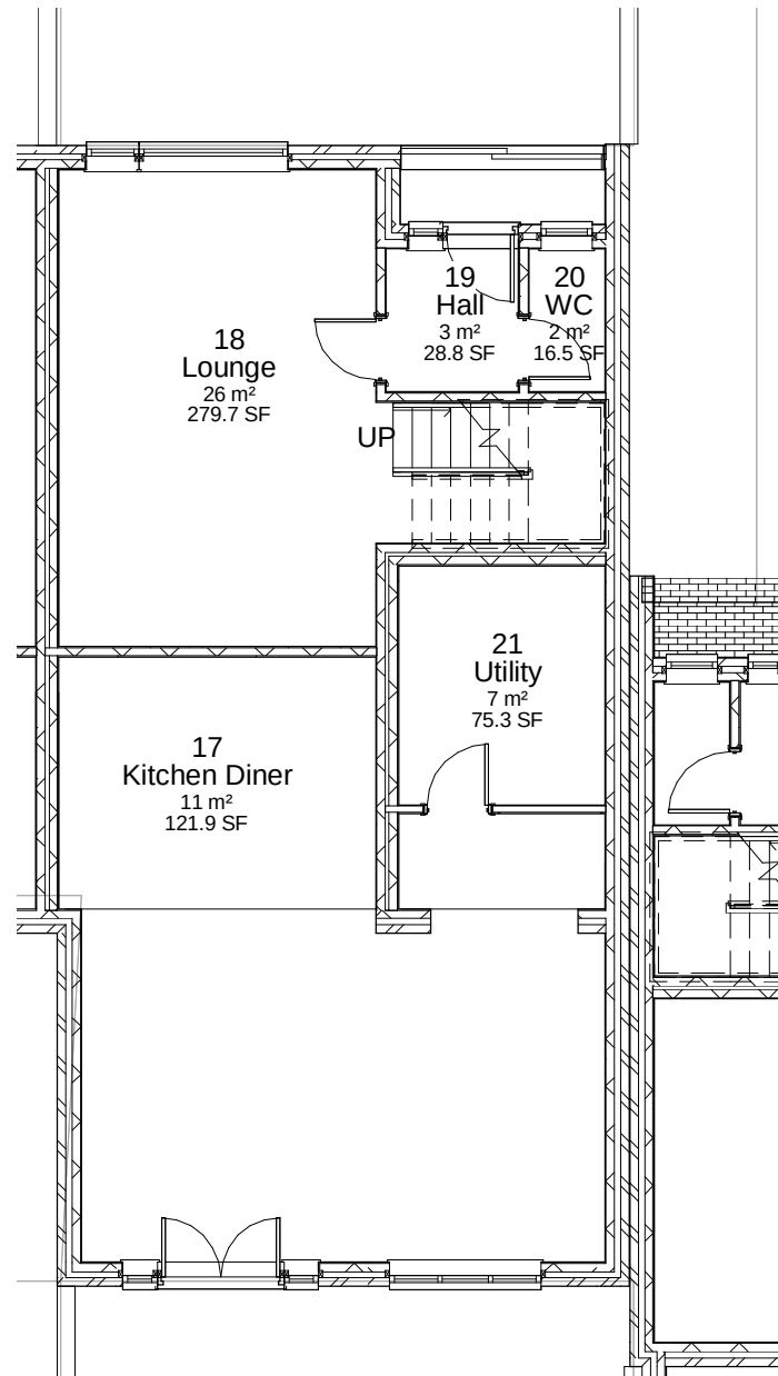
1 Ground - 40A 1 : 100
