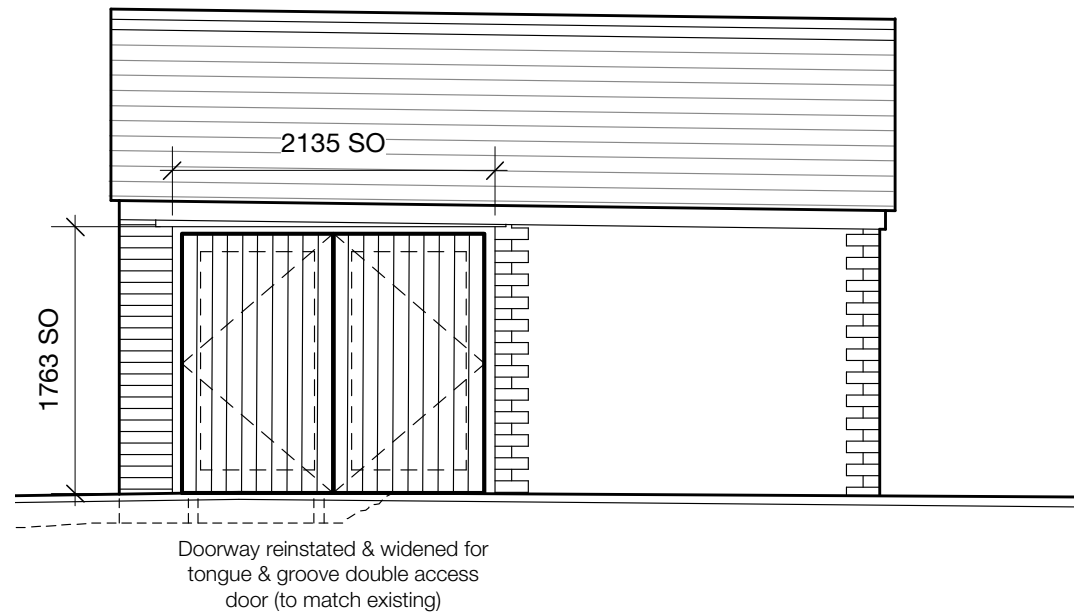
1 Woodstore - North Elevation Scale: 1:50
