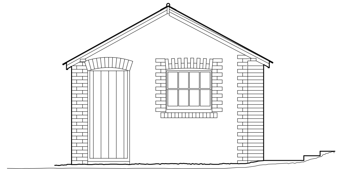
4 Woodstore - East Elevation Scale: 1:50
