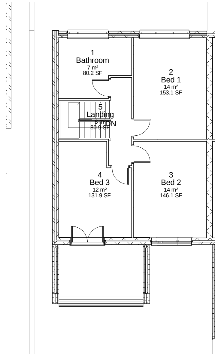
2 Level 1 - 40 1 : 100
