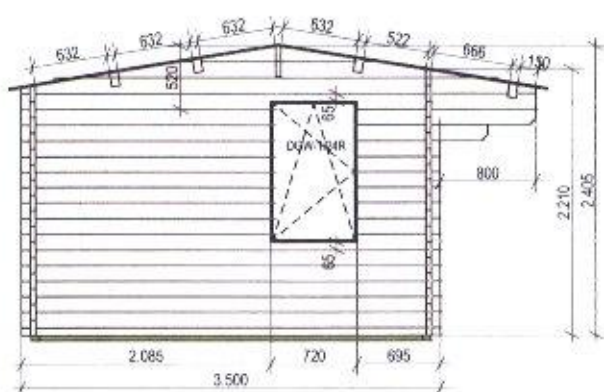
Elevation 2
