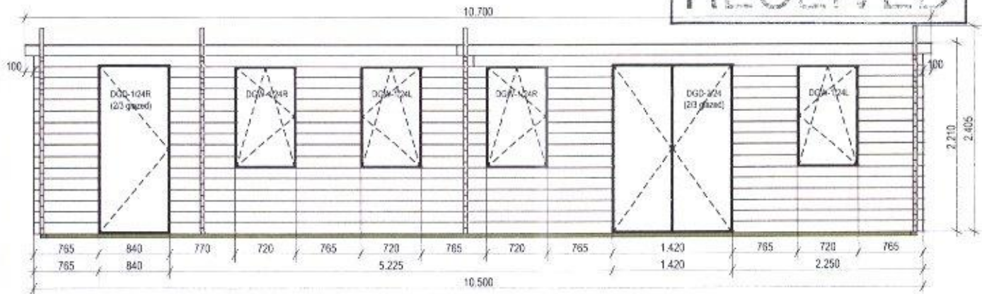
Elevation 1
