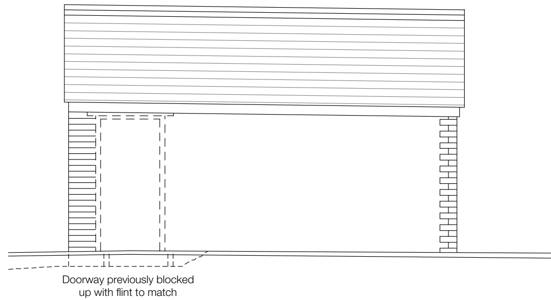
1 Woodstore - North Elevation Scale: 1:50
