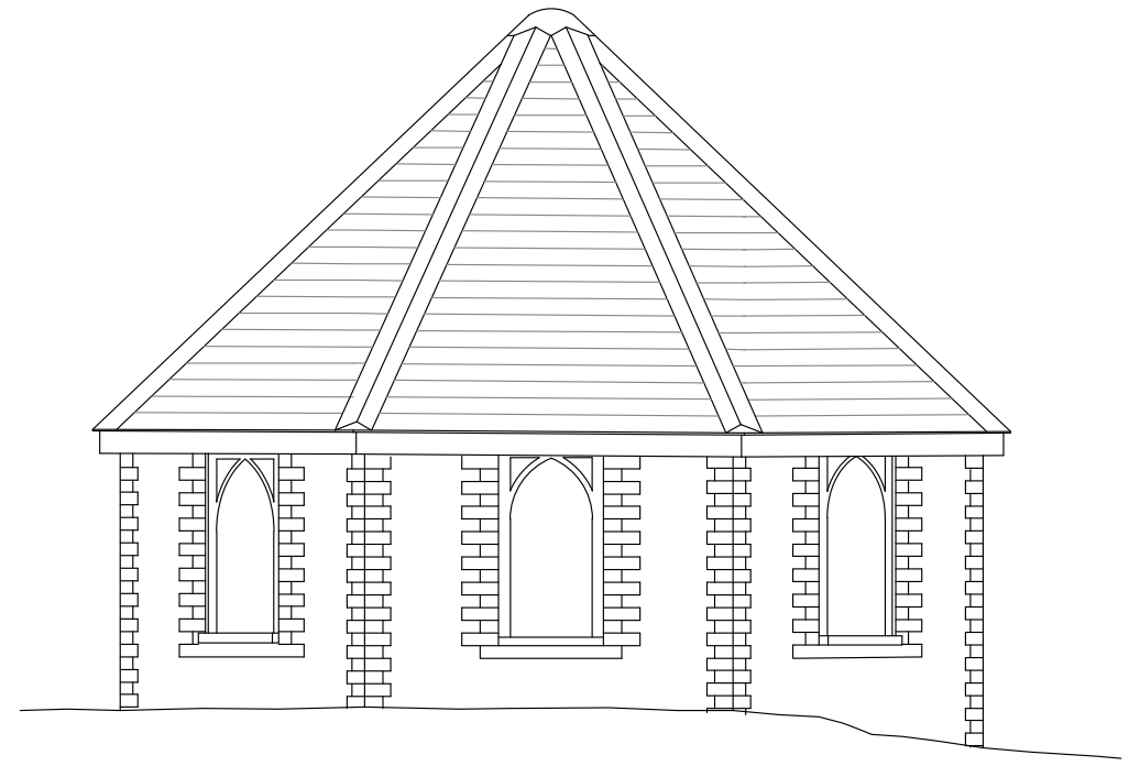
Dairy - East Elevation Scale: 1:50
