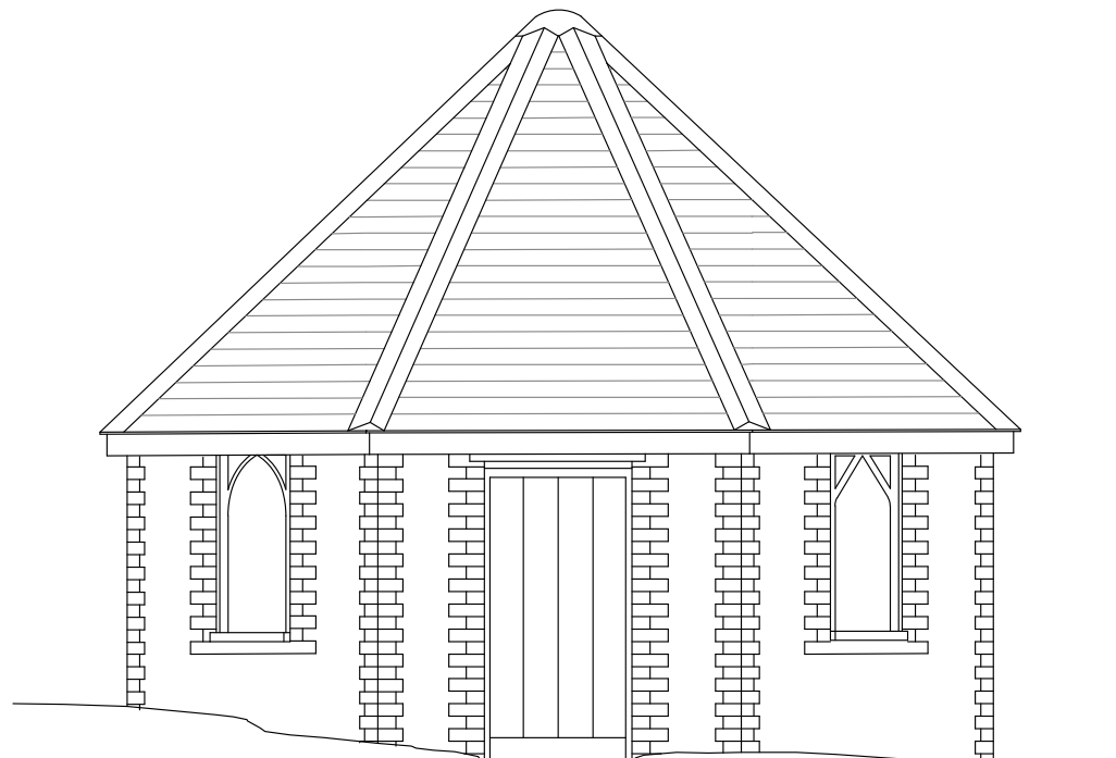
Dairy - West Elevation Scale: 1:50
