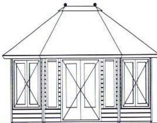
Vooraanzicht / Front view / Vorderansicht WEST ELEVATION
