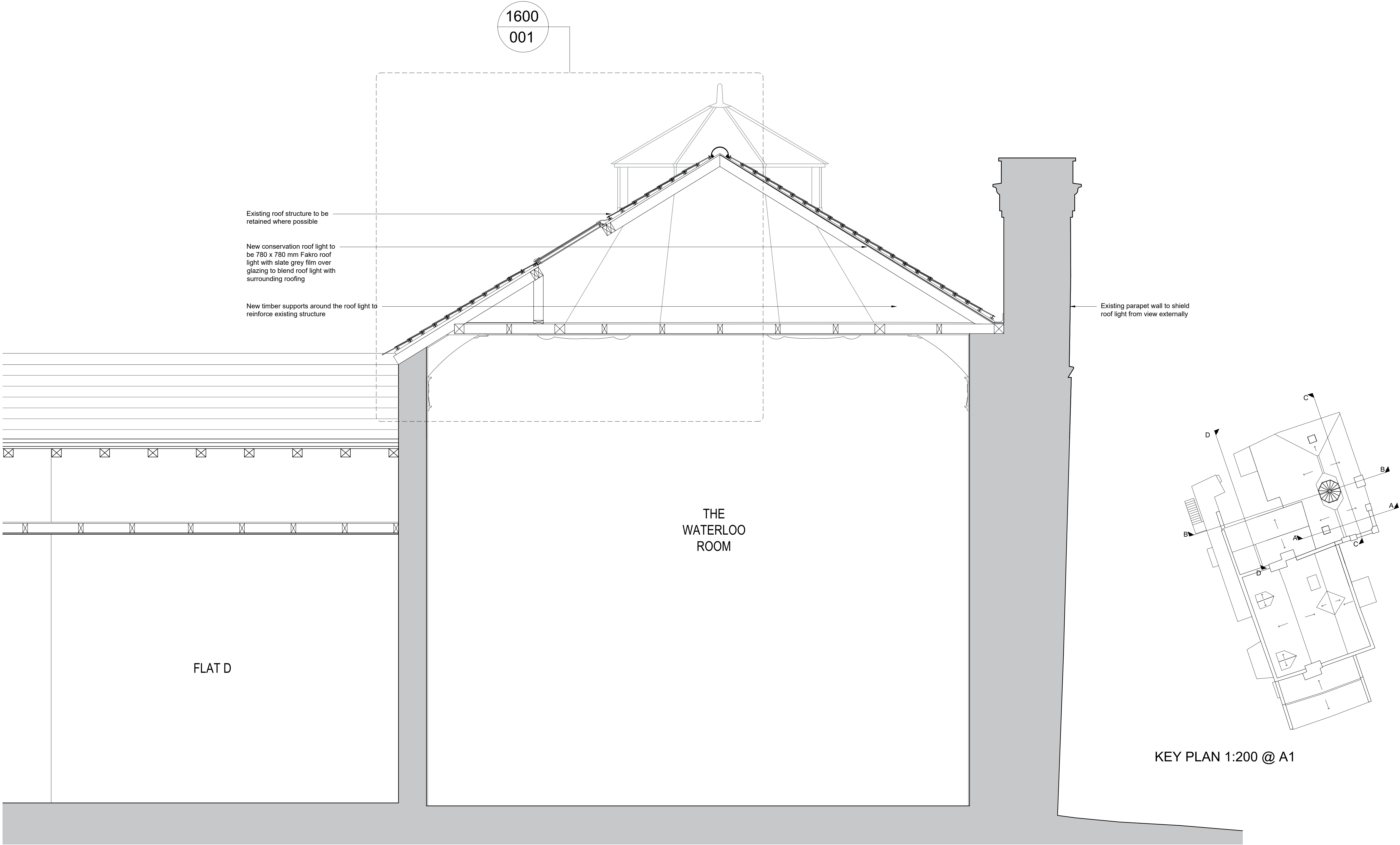
SECTION A-A 1:20 @ A1
