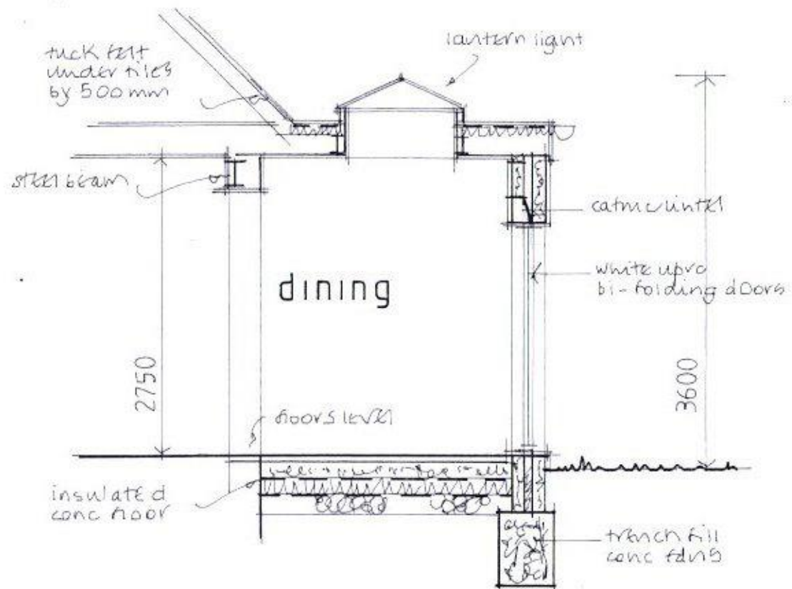
section a-a
