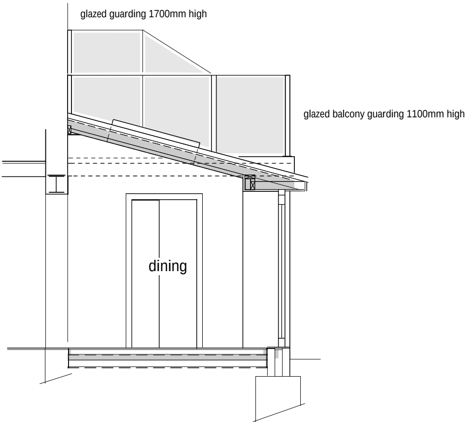
Prop. Section A - A 1 : 50 scale
