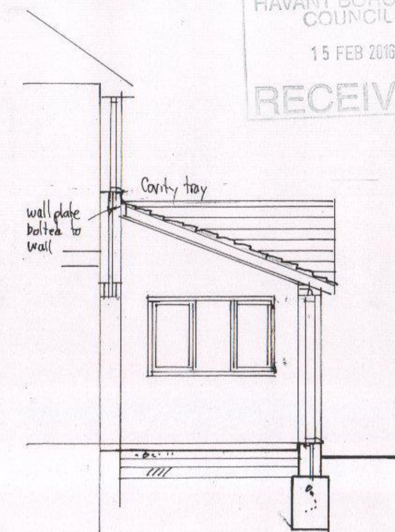
Section A-A
