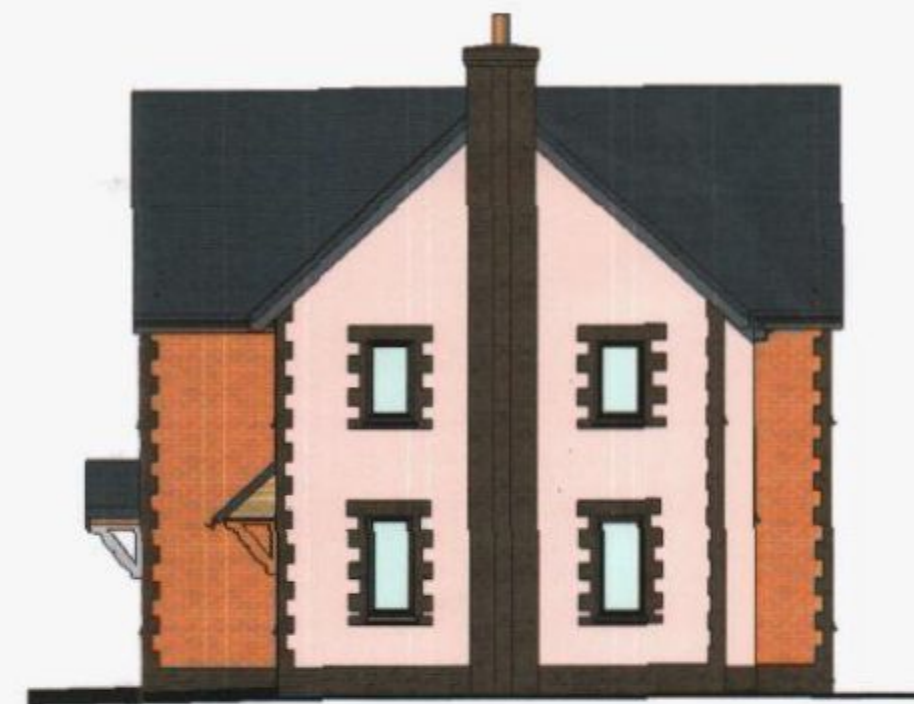
Type 4- Plots 5,6 Right Elevation 1:100
