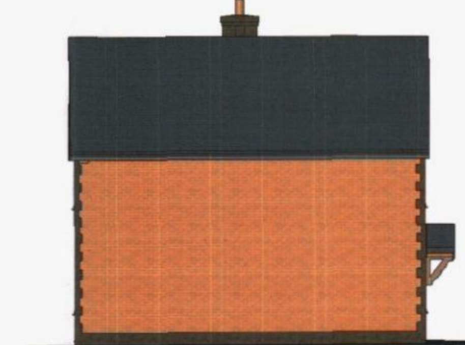
Type 4- Plots 5,6 Left Elevation 1:100
