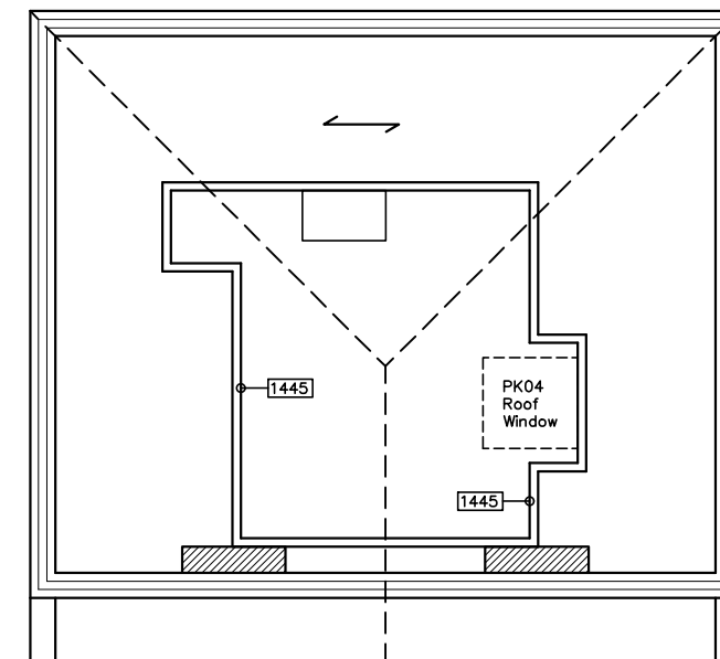
Loft Plan
