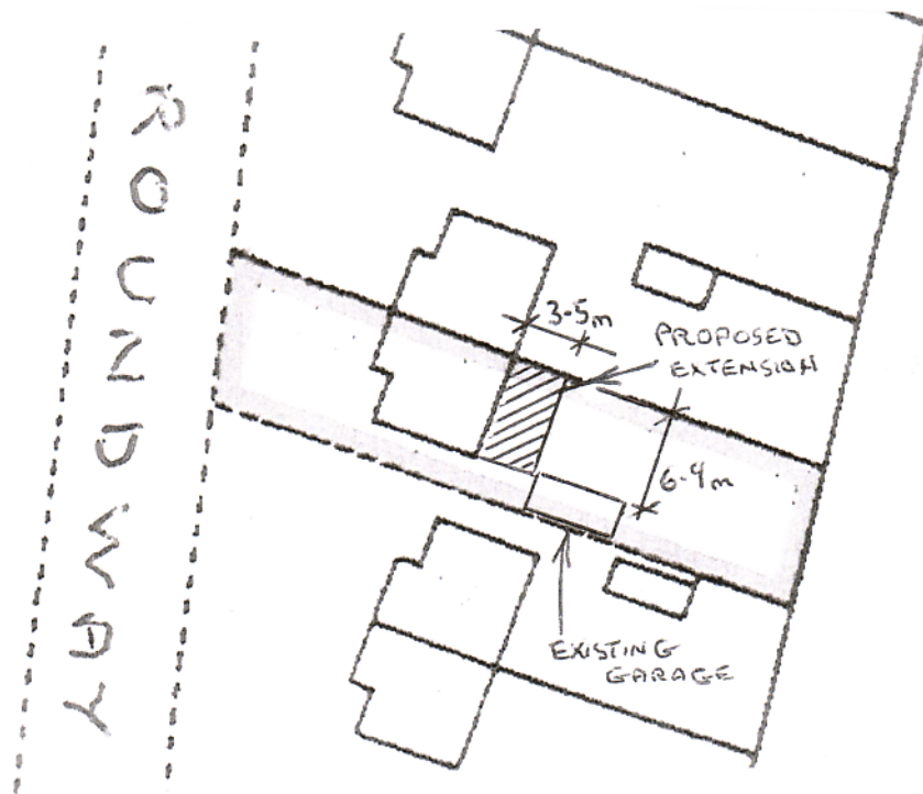
SITE PLAN 1:500
