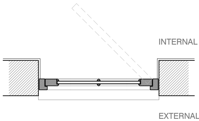
PLAN 1:20
