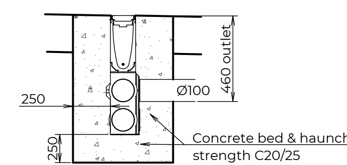
ACO MULTIDRAIN UNIVERSAL SUMP 1:20
