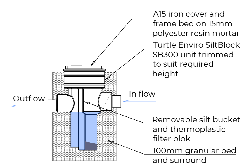
TURTLE ENVIRO SILTBLOK SB300 SILT TRAP 1:20
