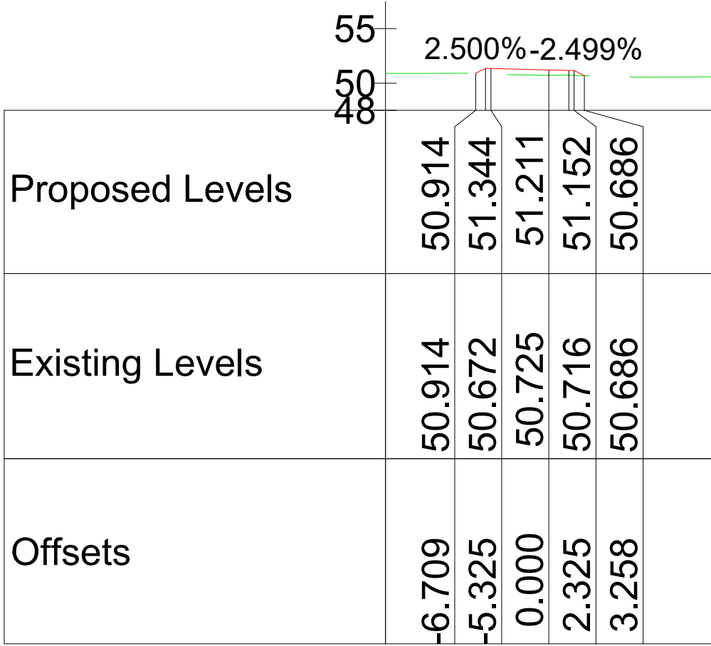
Chainage 1140.000
