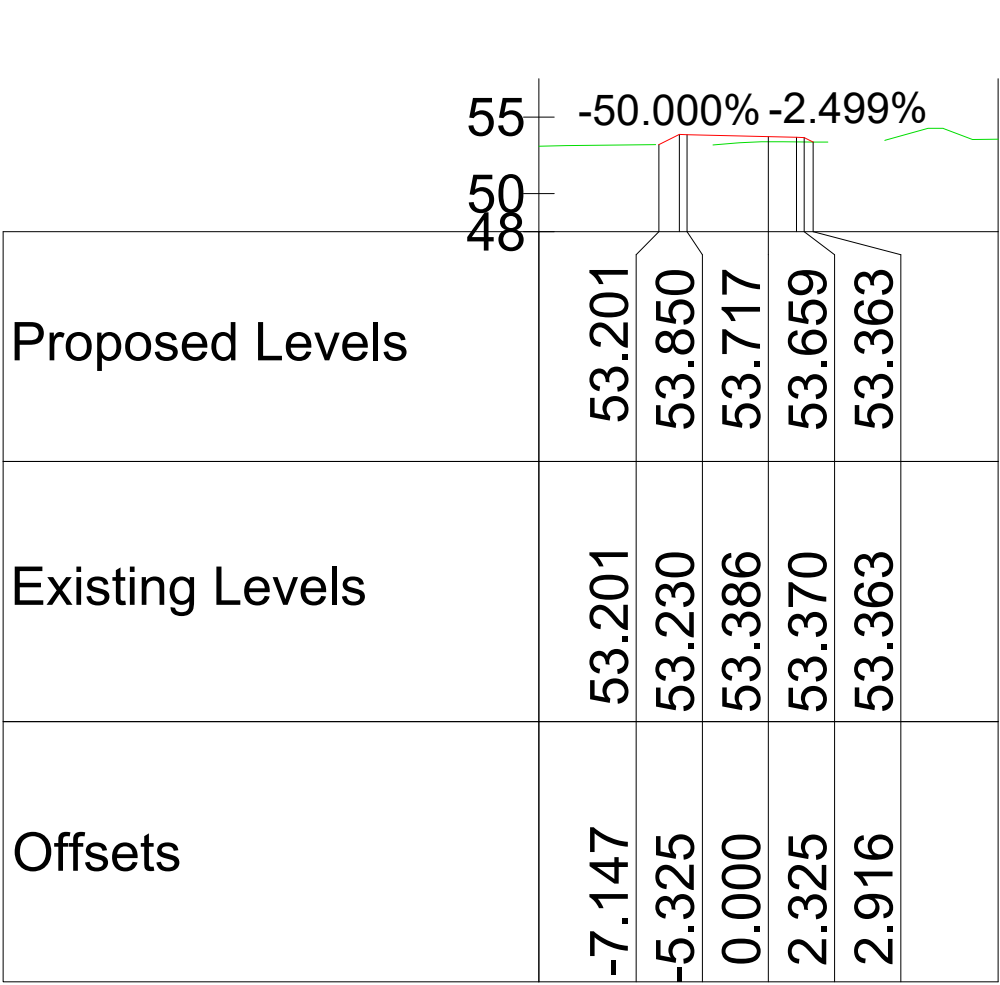
Chainage 1040.000
