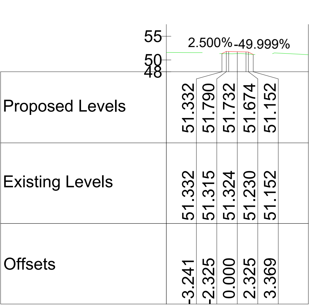
Chainage 1100.000
