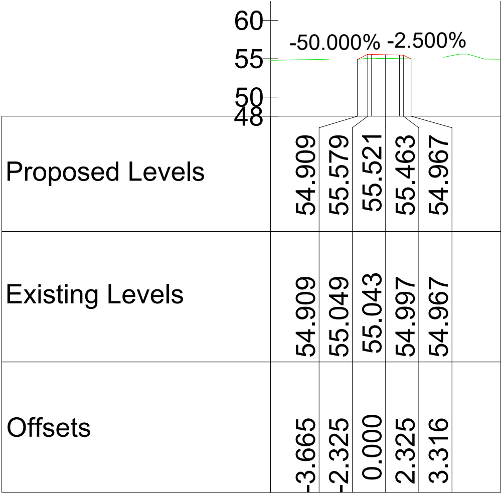
Chainage 980.000
