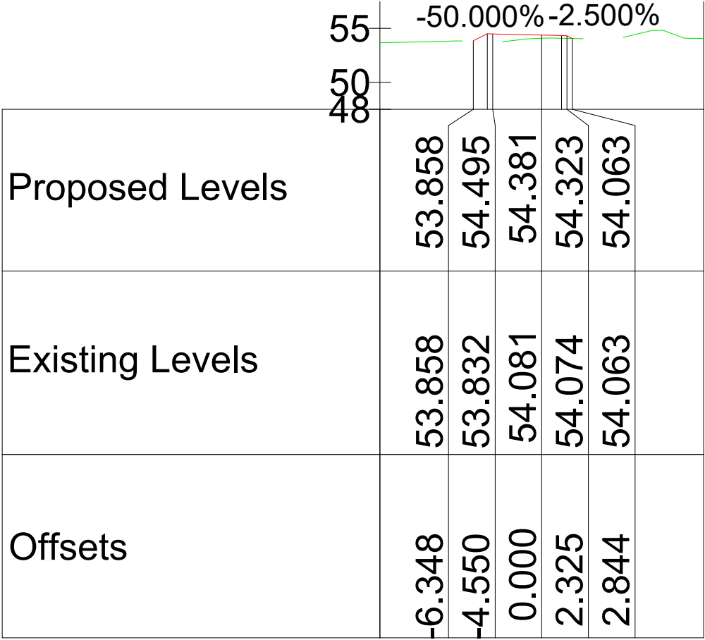
Chainage 1020.000
