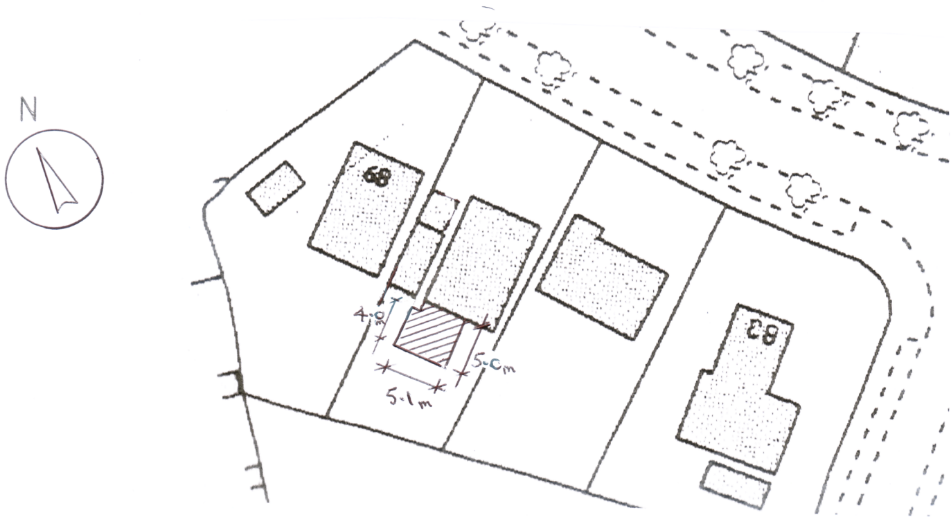
SITE PLAN 1:500
