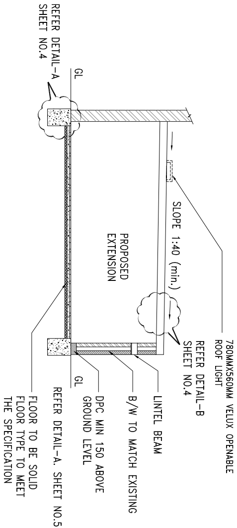
2 SECTION A-A SCALE 1:100
