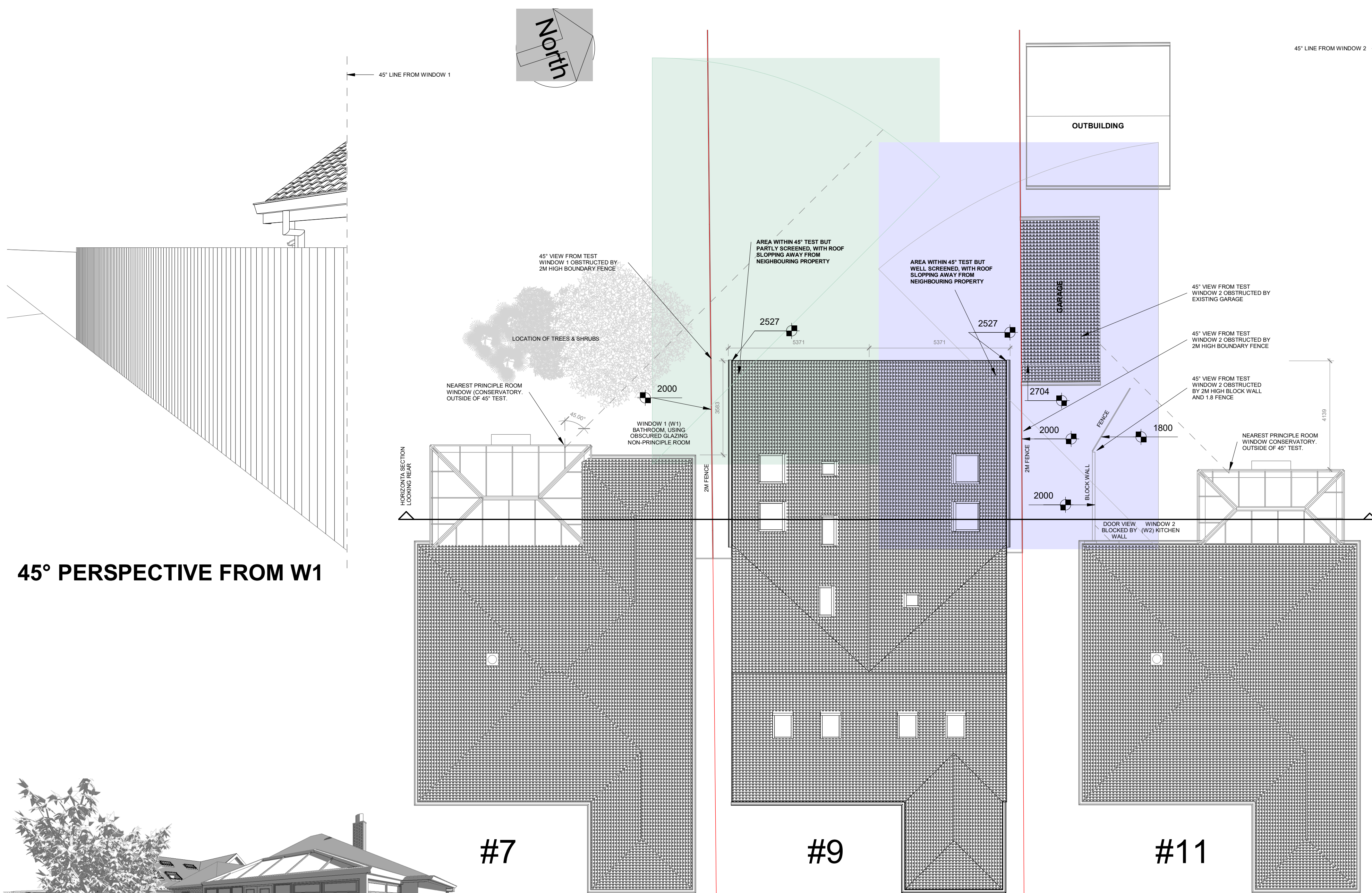
45° TESTING 1 : 100
