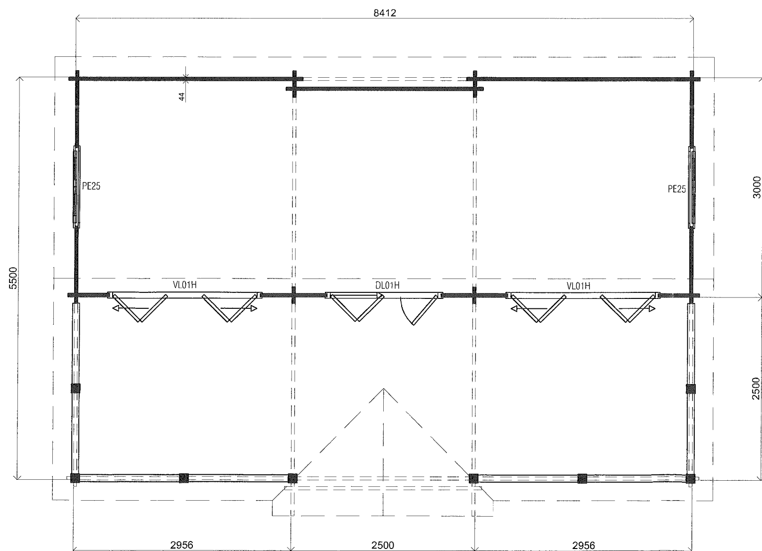
Plattegrond / Plan
