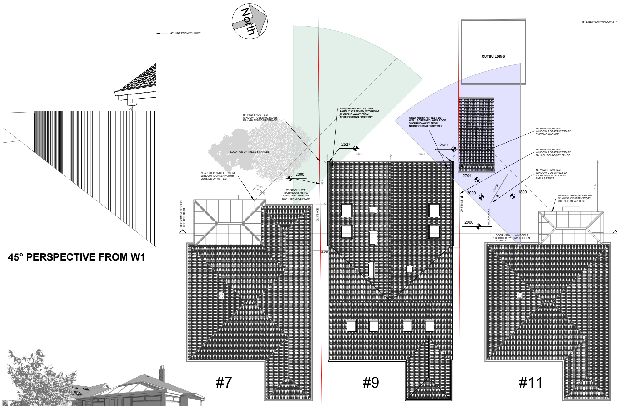
45° TESTING 1 : 100
