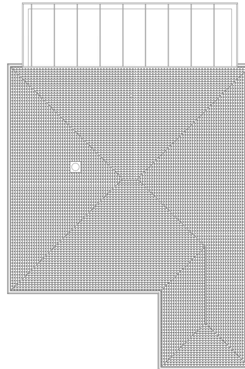
ROOF PLAN 1 : 100
