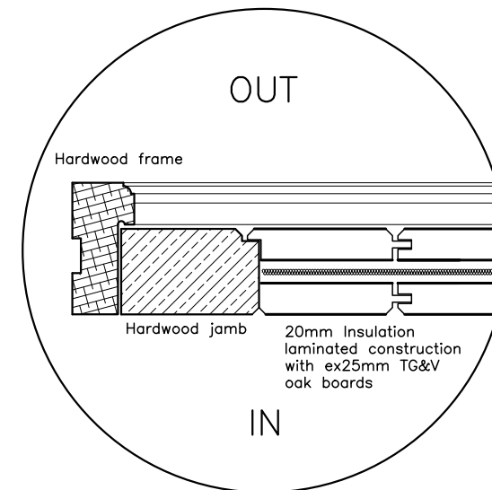
Jamb
