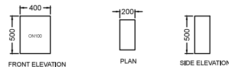
PURIFIED AIR O.N.100 ODOUR CONTROL UNIT
