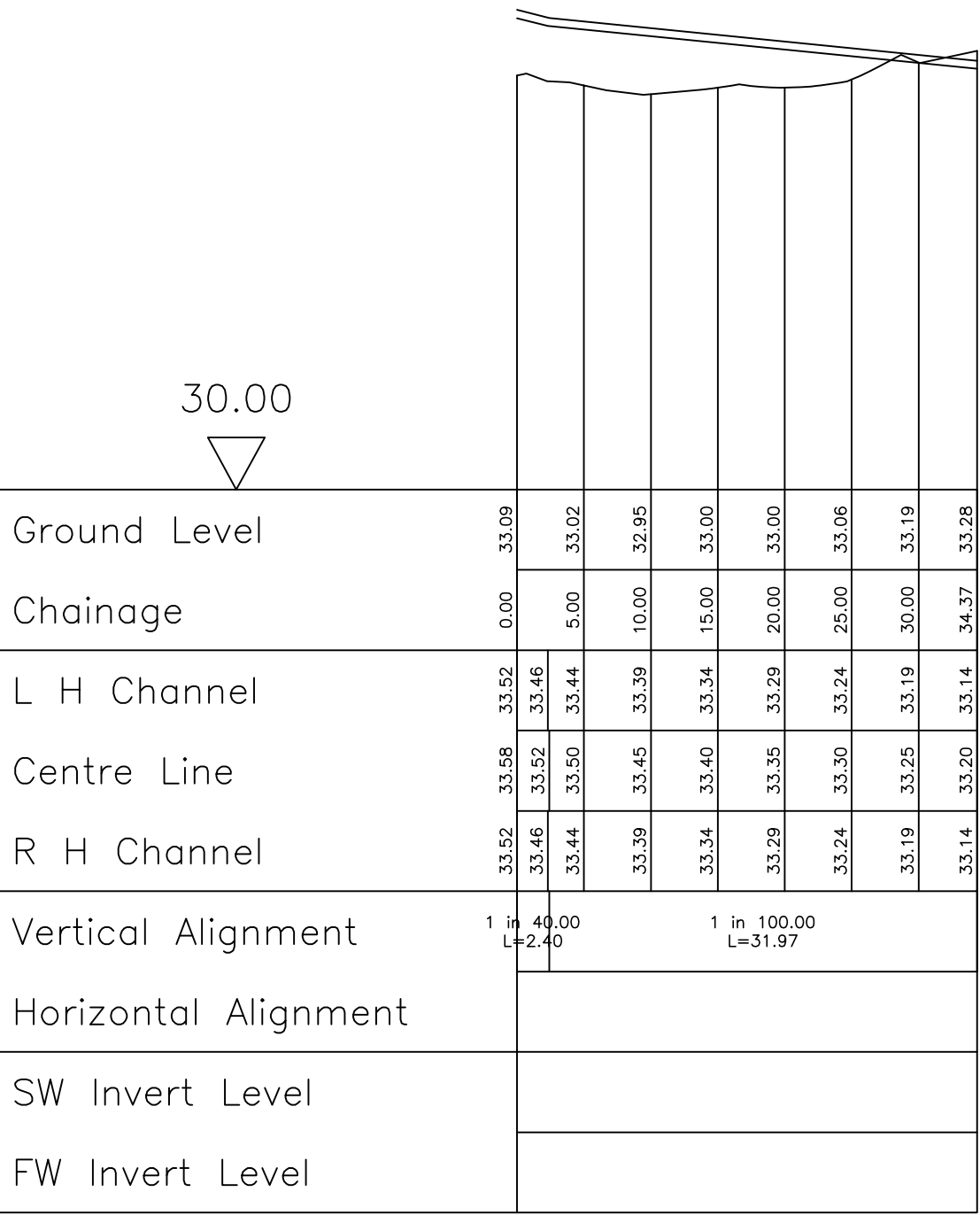
Road 3 Horiz. 1:500 Vert. 1:50
