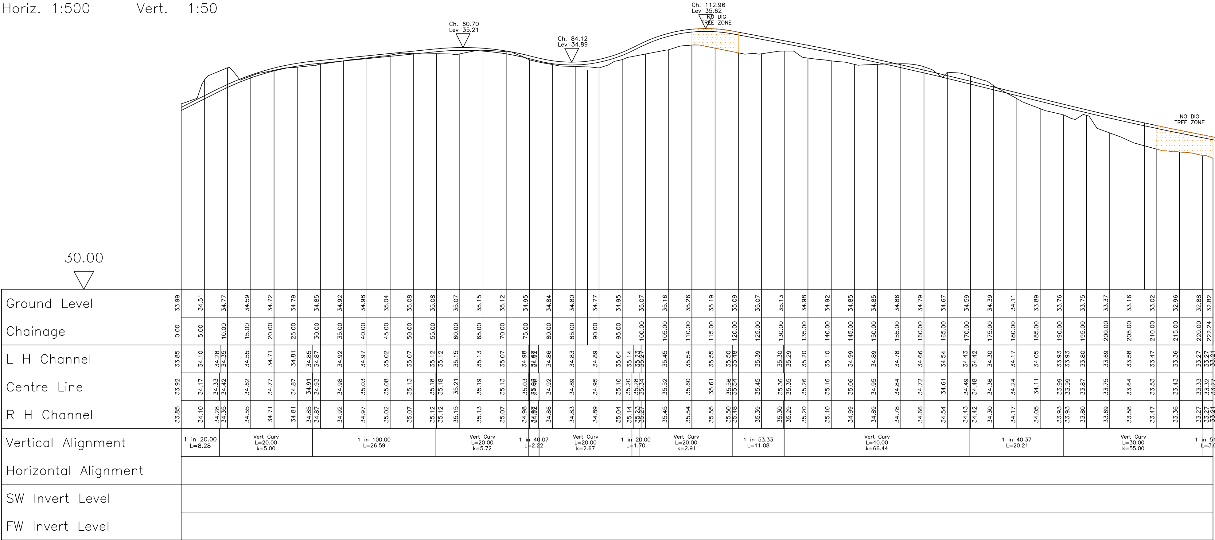
Road 2 Horiz. 1:500 Vert. 1:50
