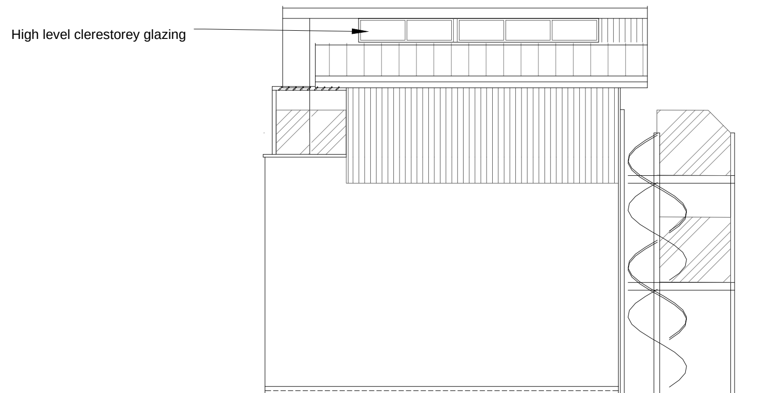
SIDE (SW)
