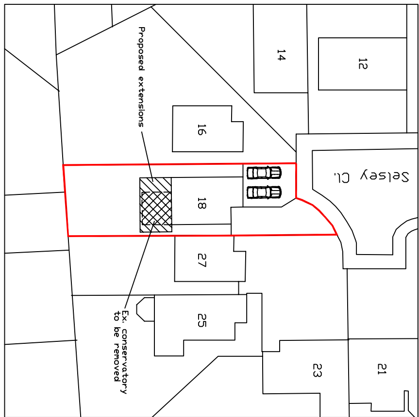
SITE PLAN 1:500
