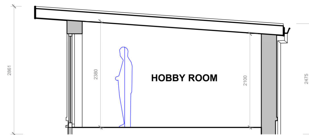
CROSS SECTION 3 1 : 50
