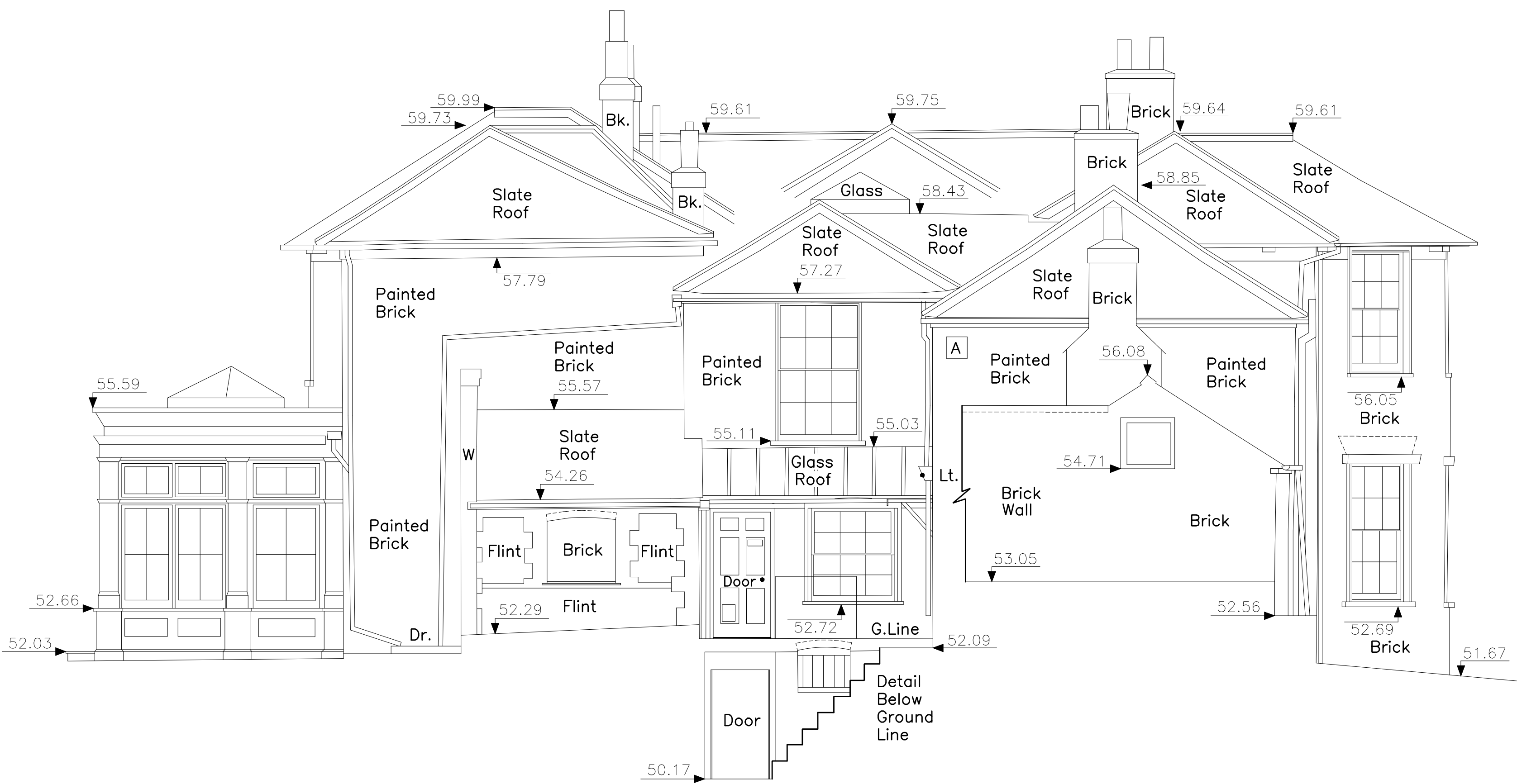
ELEVATION 4
