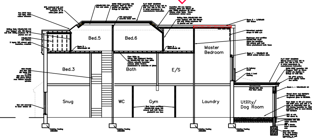
SECTION D-D
