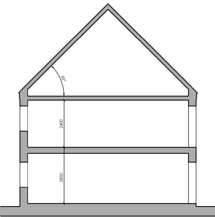
FLATS - SECTION
