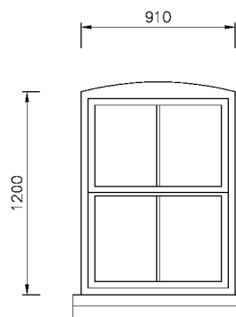
Elevation
