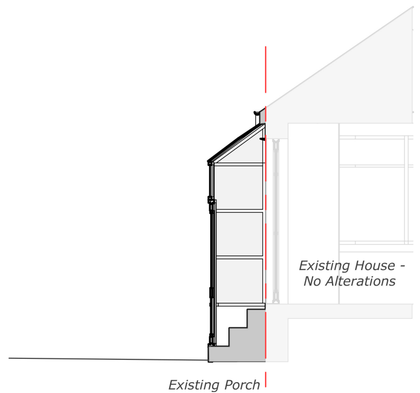
Existing Section A-A 1:50
