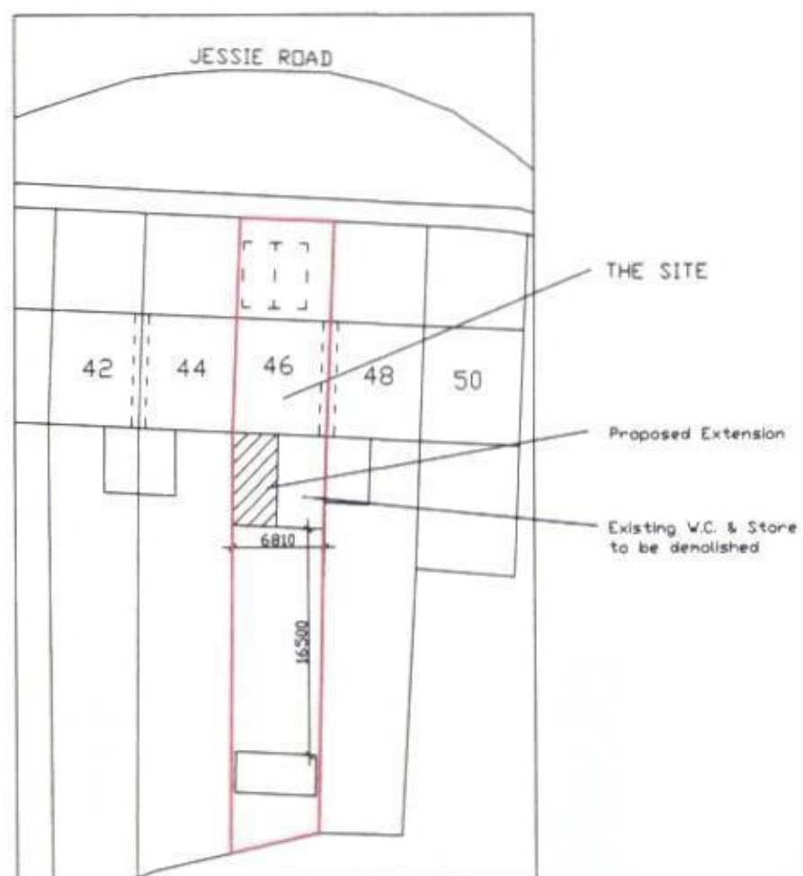
SITE PLAN 1:500
