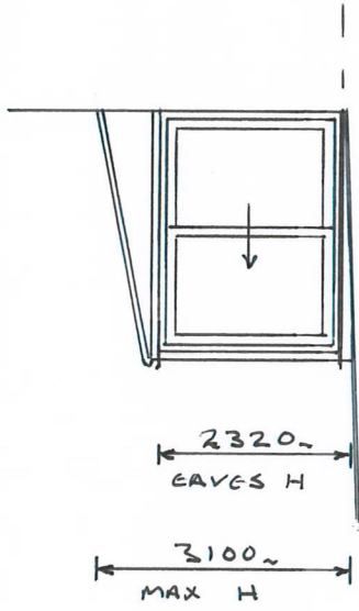
RIGHT ELEVATION
