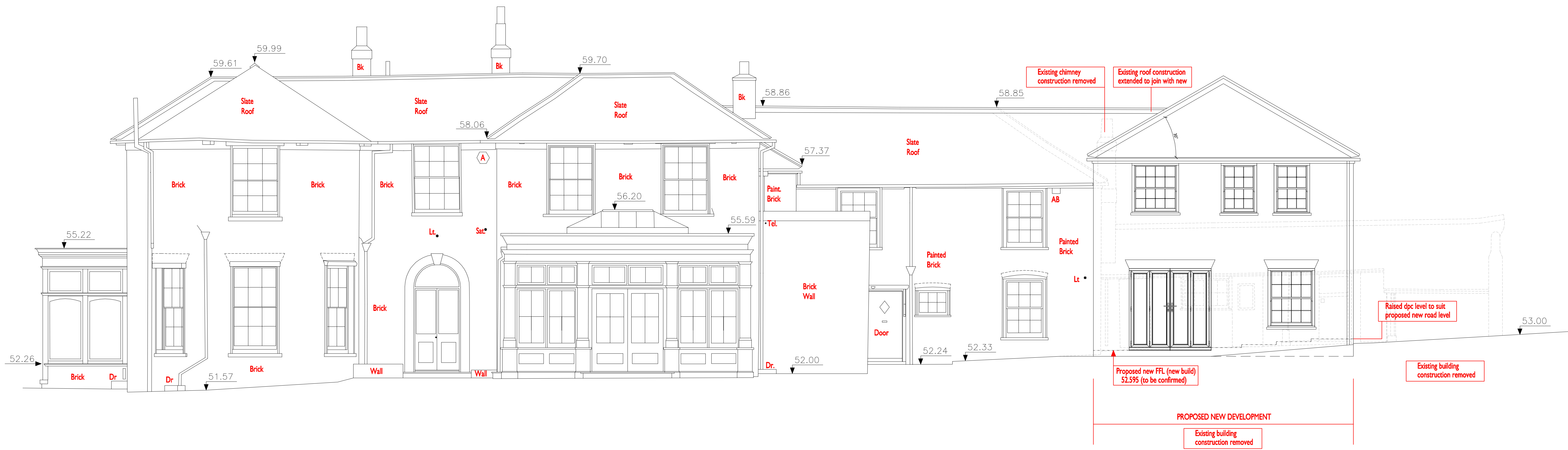
ELEVATION 3
