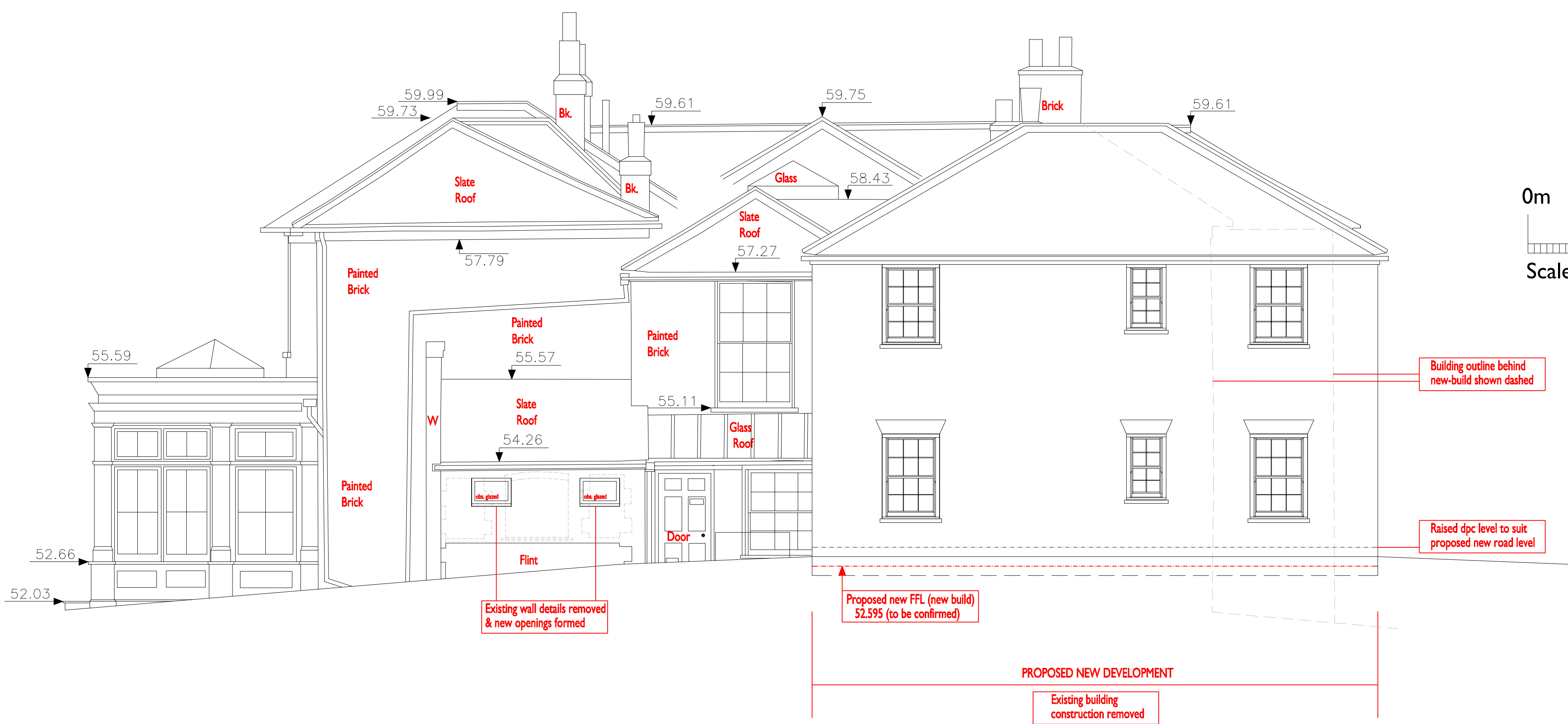
ELEVATION 4
