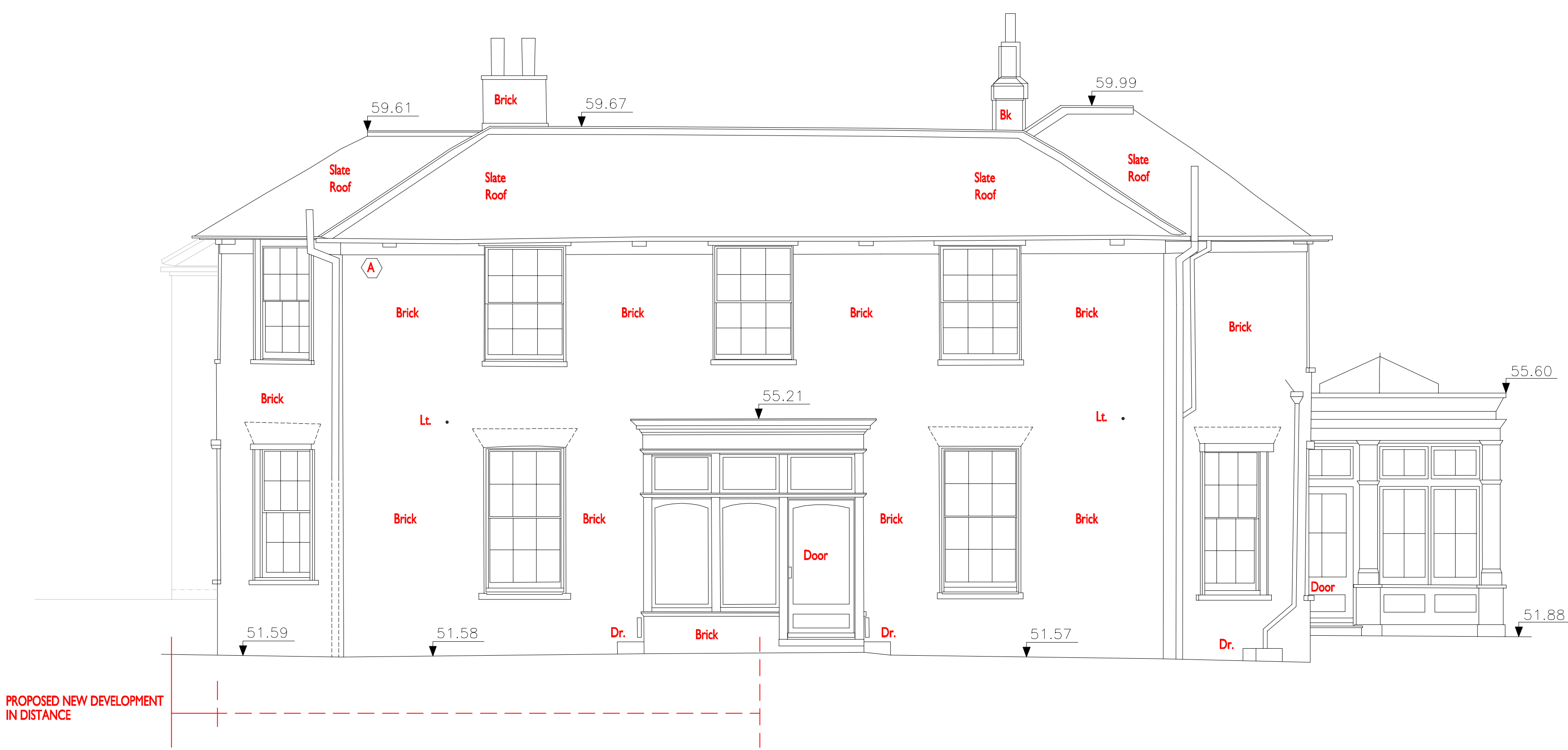
ELEVATION 2
