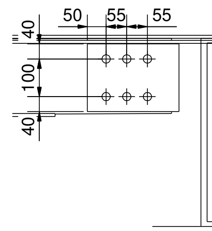
K - K 1:10
