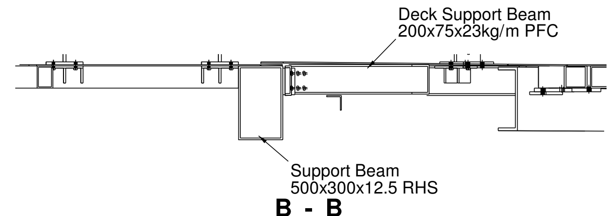
B - B 1:25
