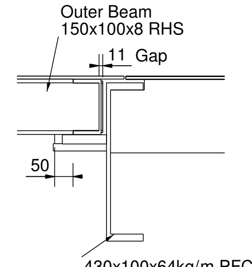
D - D 1:10
