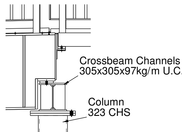
F - F 1:25
