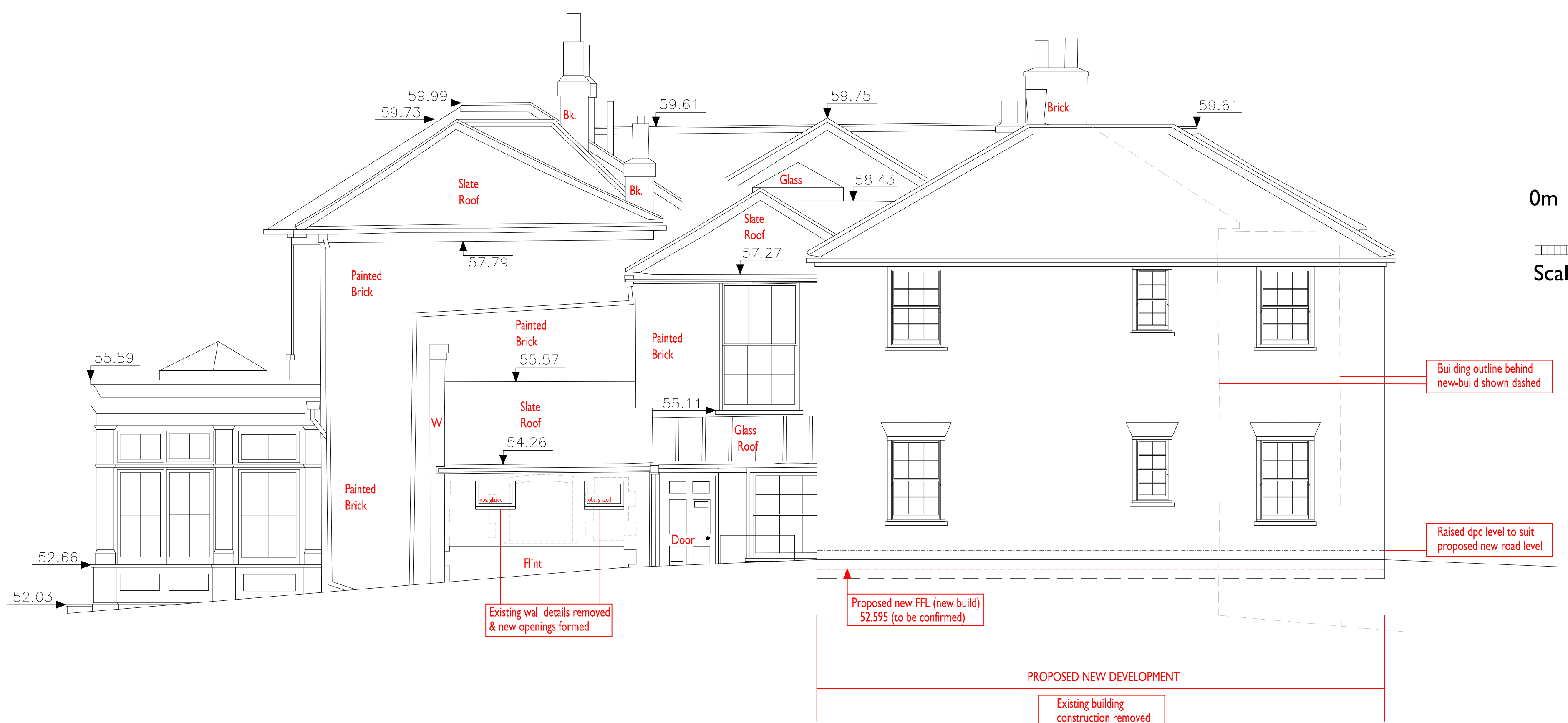
ELEVATION 4
