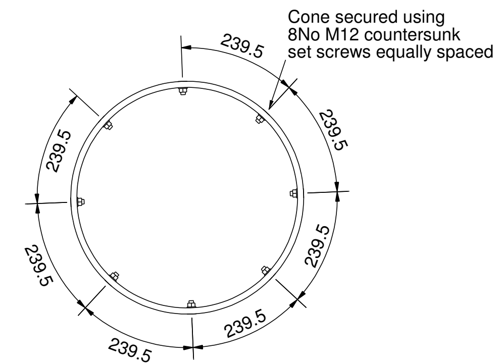
D - D 1:10
