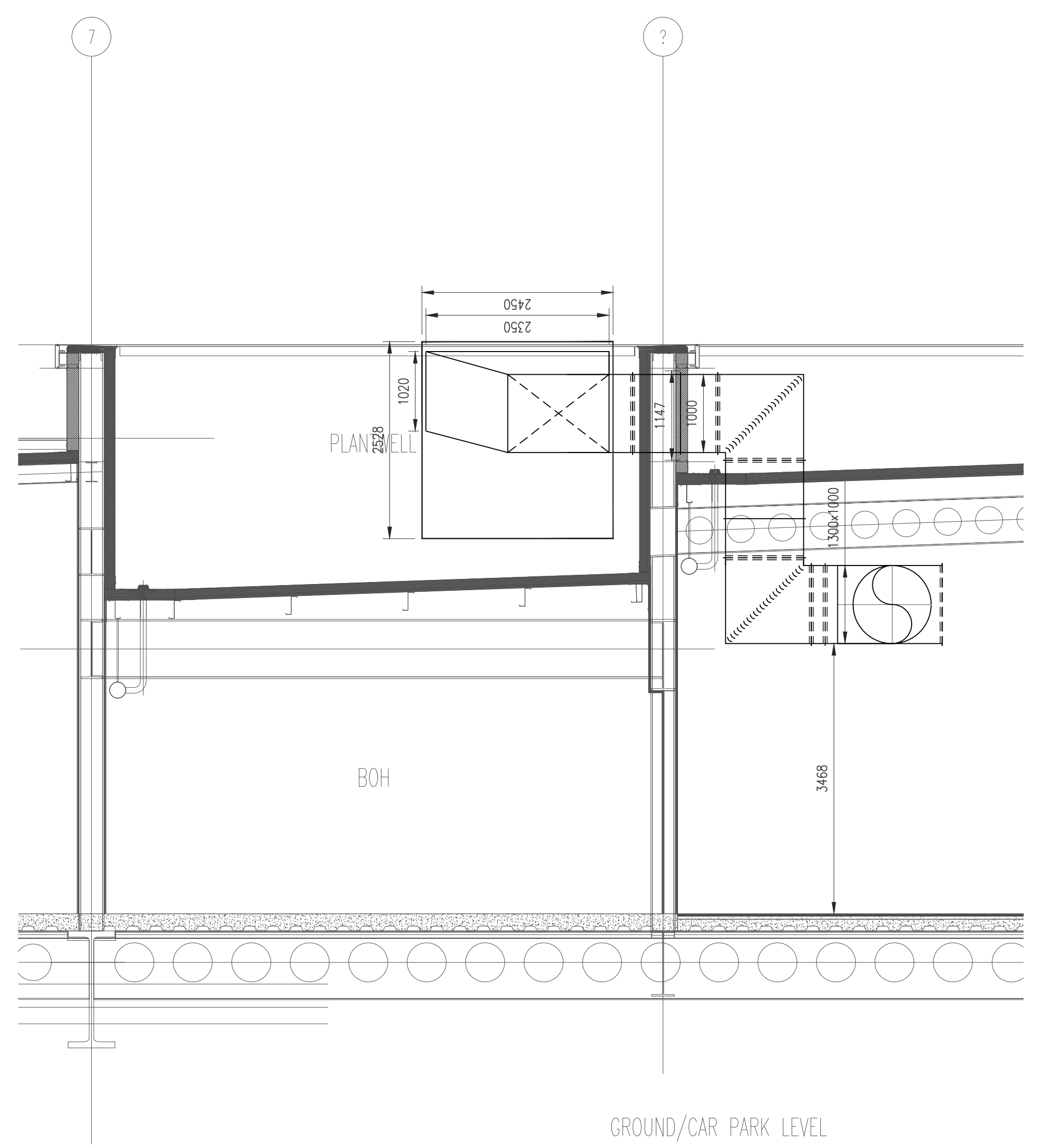
SECTION A-A
