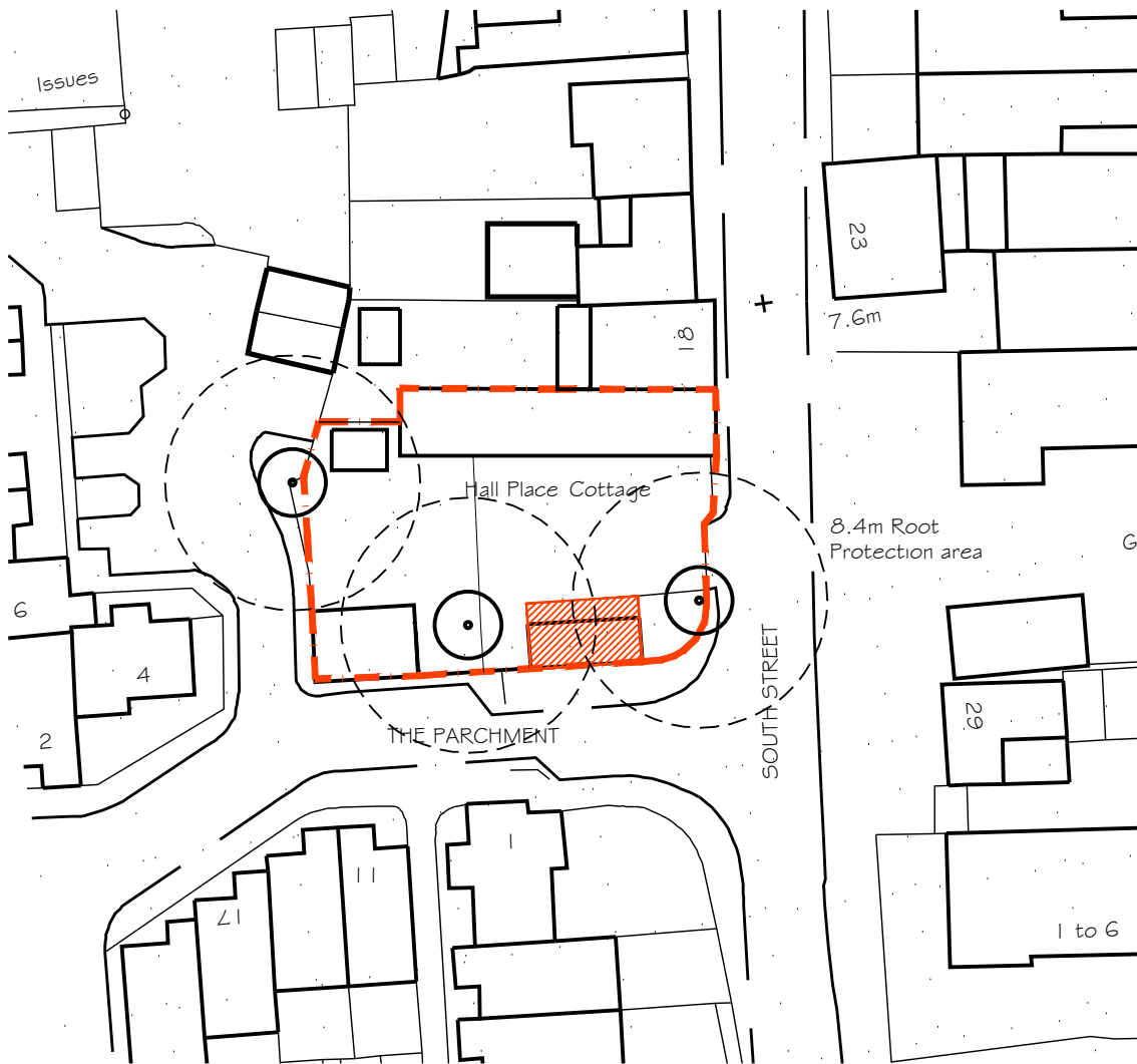
Block Plan 1 : 500
