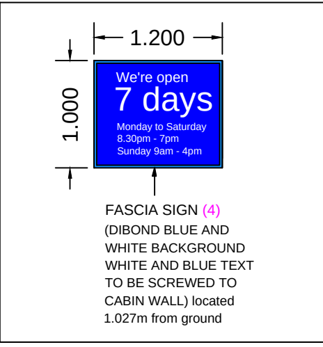
FASCIA SIGN 1:50 @ A3
