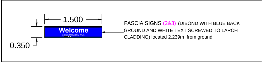
FASCIA SIGN 1:50 @ A3
