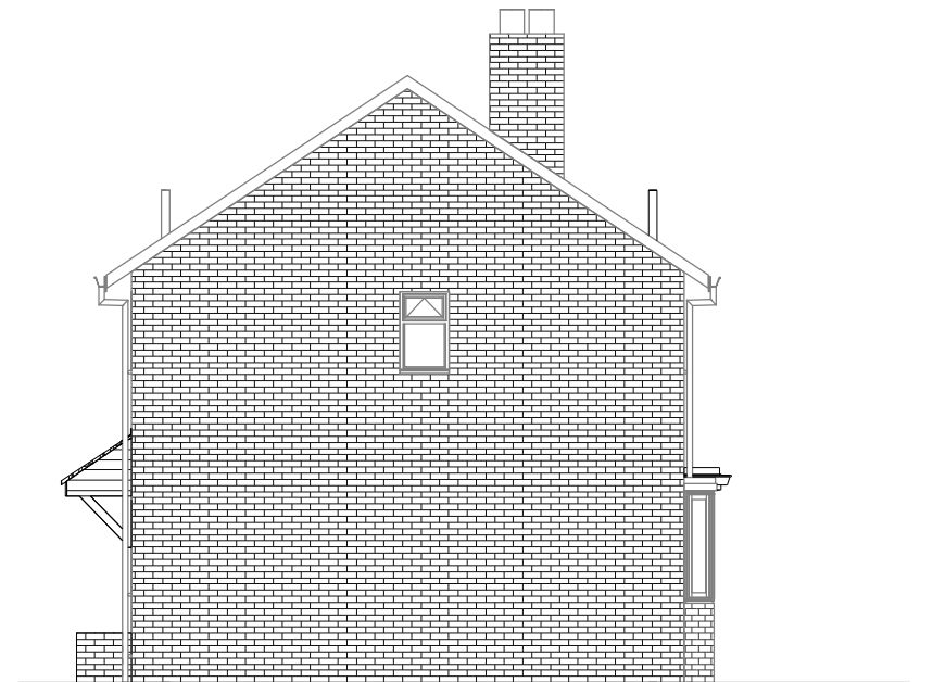
WEST 1 : 100
