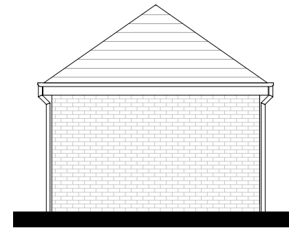
5 Gable 1 1 : 100
