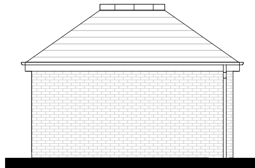
4 Rear 1 : 100
