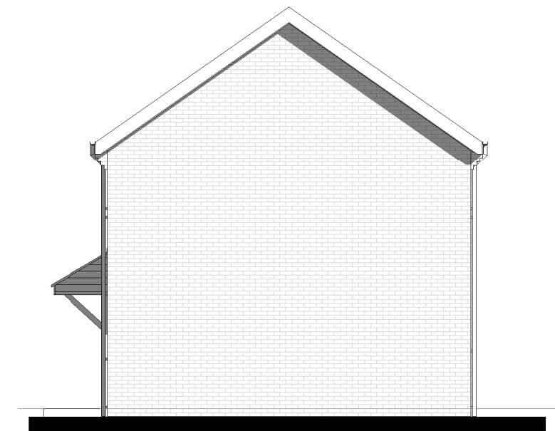
2 Gable 1 1 : 100
