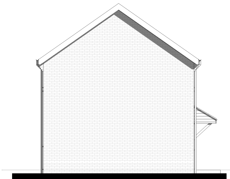
4 Gable 2 1 : 100
