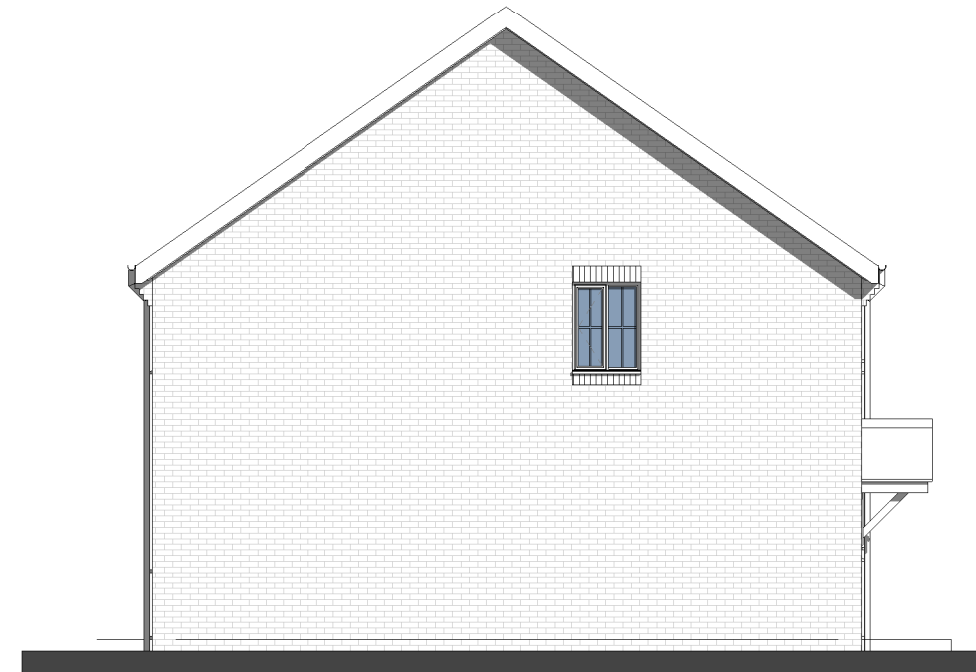
4 Gable 2 1 : 100
