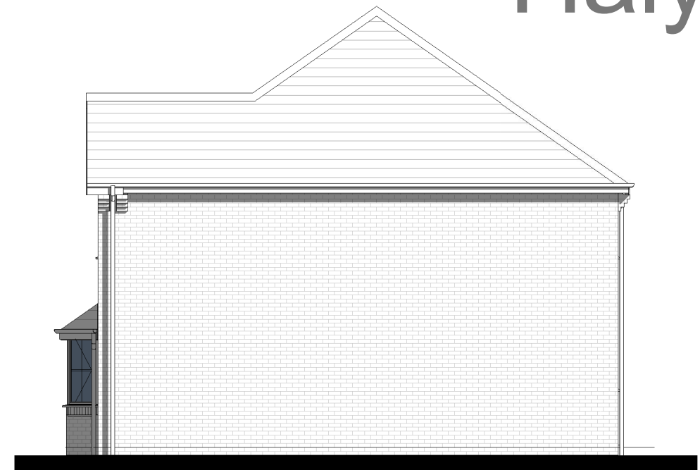
2 Gable 1 1 : 100
