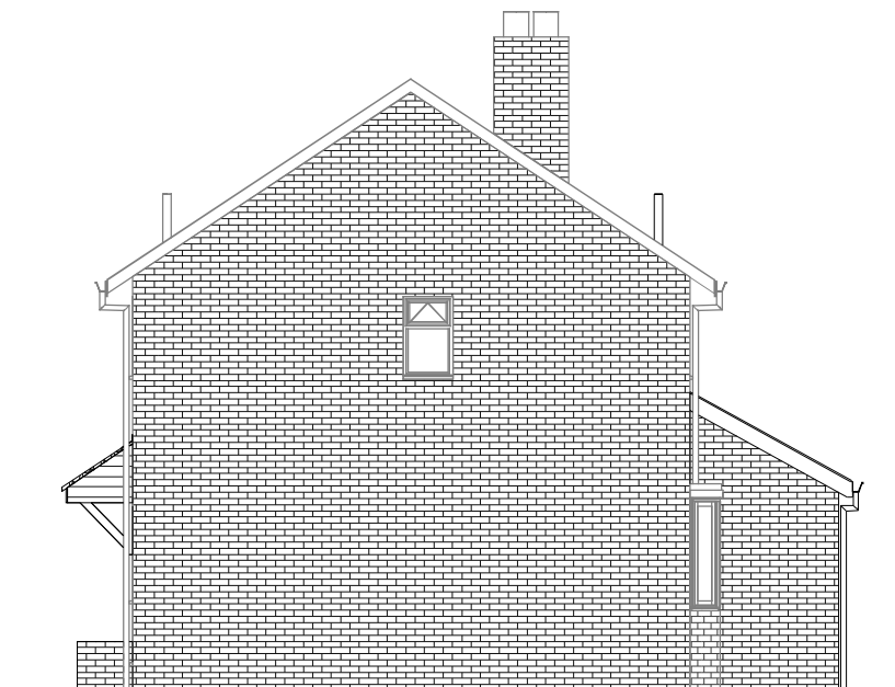
WEST 1 : 100
