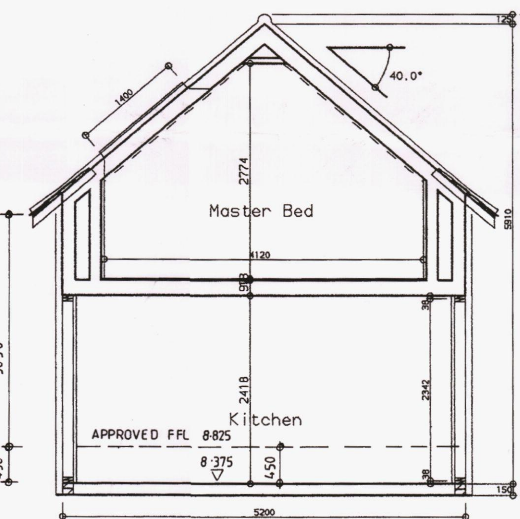
Section D-D
