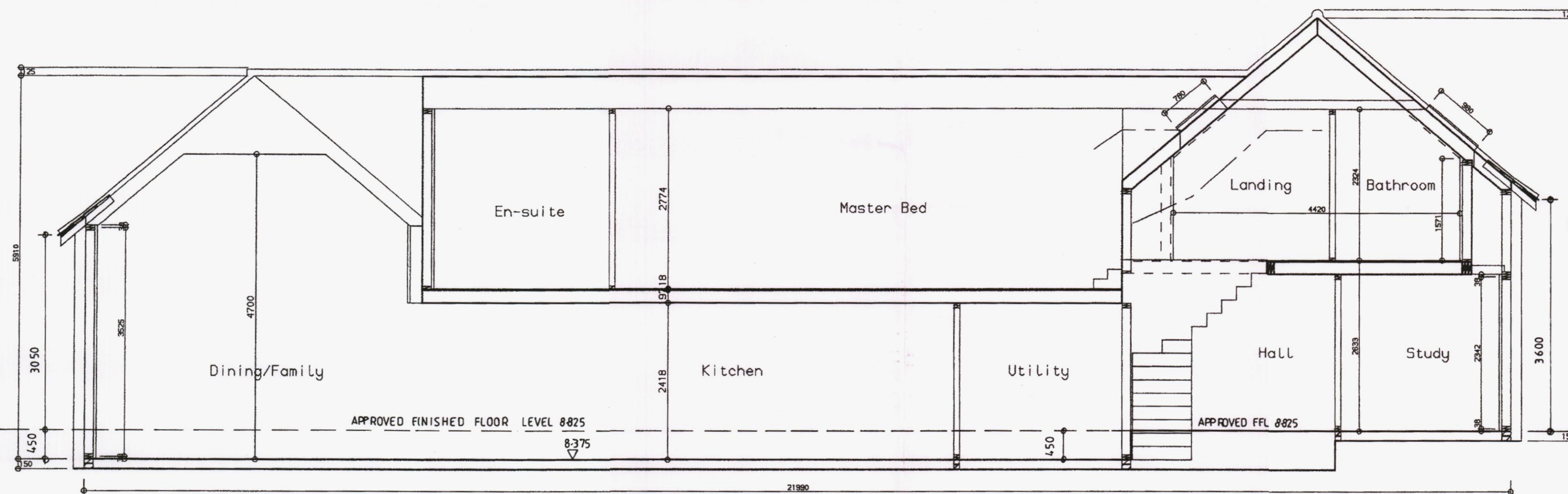
Section A-A
